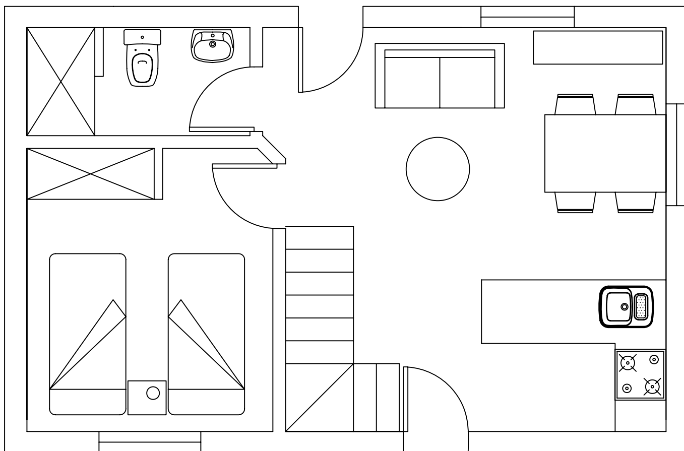
PLANTA BAJA
